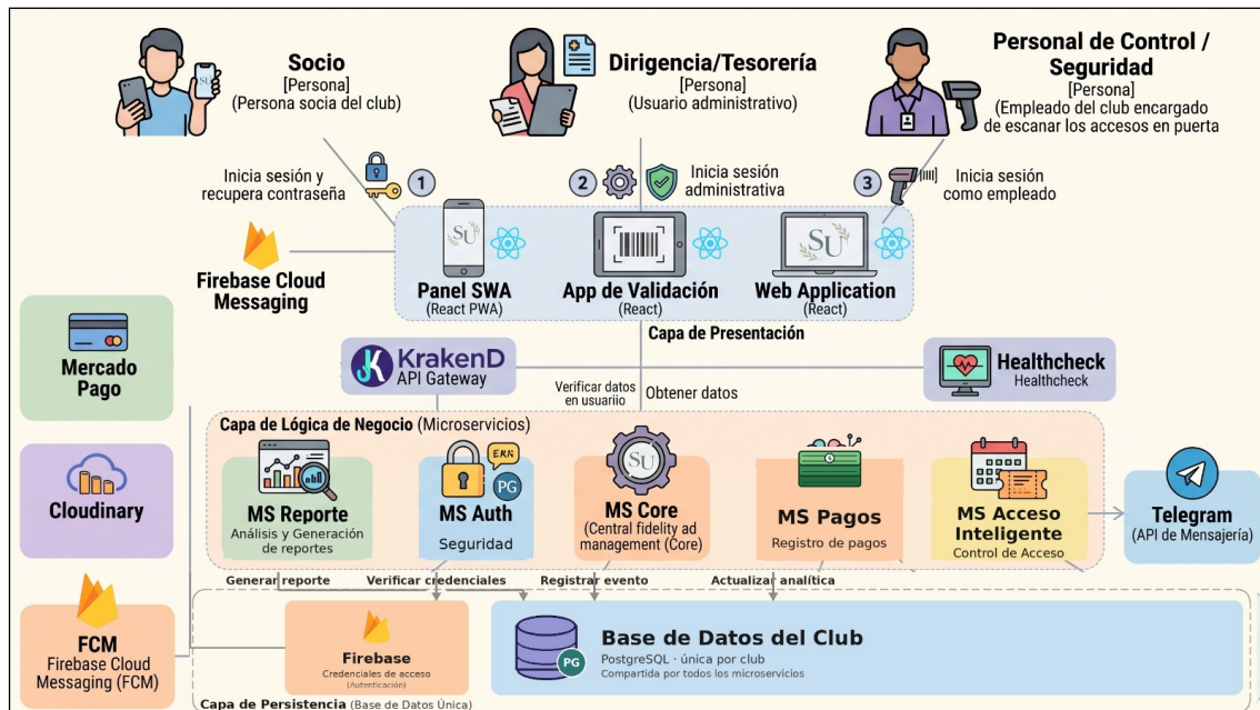
Figura 17: Diagrama de contenedores (C2) que detalla el aislamiento de las interfaces de front-end respecto a los microservicios y bases de datos transaccionales.
