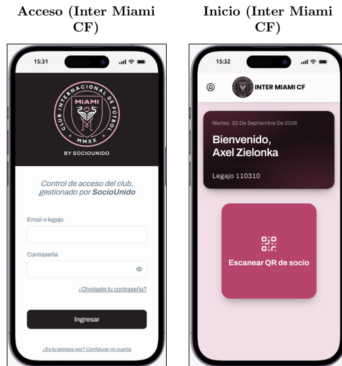
Figura 13: Pantallas de acceso y menú principal de la App para Empleados.
